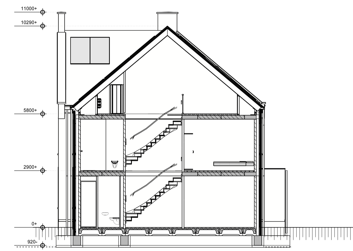
Doorsnede
